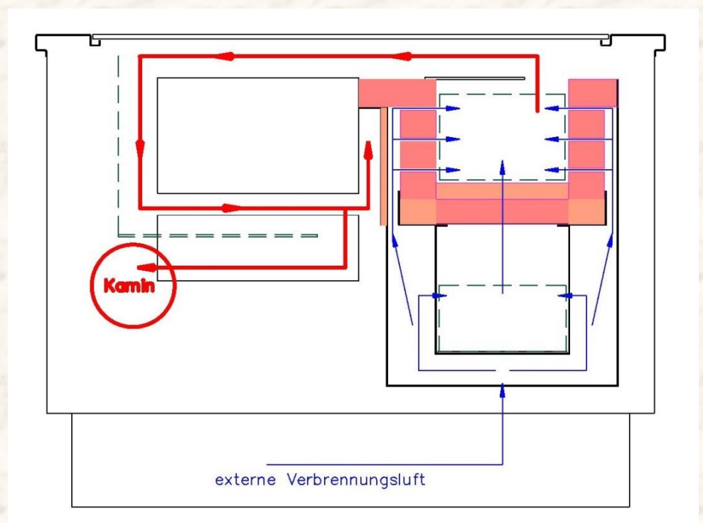
schematische Darstellung vom Brennraum
